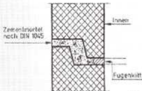
Bild 2.3-78 Schachtringabdichtungen mit Zementmörtel (über dem Grundwasser) nach ATV A 241
