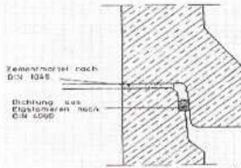
Bild 2.3-81 Schachtringabdichtung mit Olettring [404]
