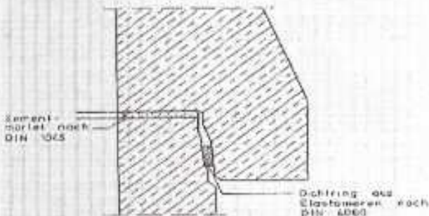
Bild 2.3-80 Schachtringabdichtung mit Röllring [404]
