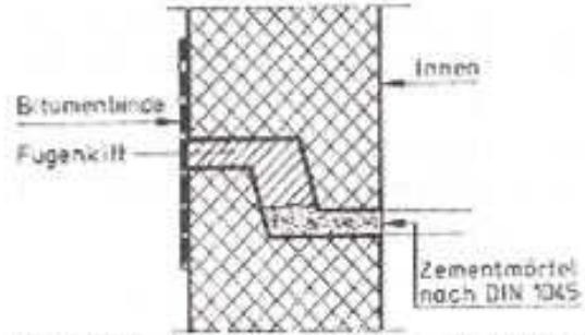
Bild 2.3-79 Schachtringabdichtung mit plastischen Dichtmitteln (im Grundwasser) nach ATV A 241
